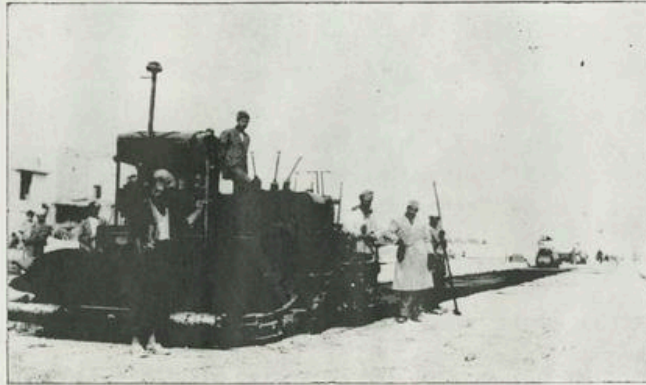
جاده میدان هراتی در حال قیر ریزی با ماشین هموار کننده اسفلت
